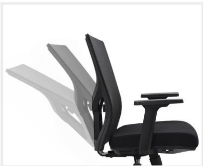
MECANISMO Syncro con 1 posición de bloqueo, control de tensión mediante perilla y slider GB.
